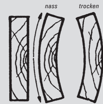
Verformungen bei einem Seitenbrett
