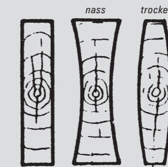
Verformungen bei einem Kernbrett
